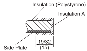
B - B
